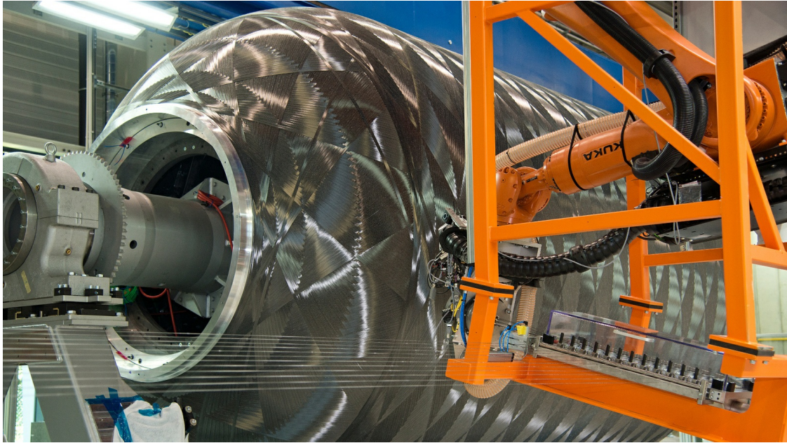
Abbildung 1: Das Boostergehäuse aus Carbonfasern für die Ariane 6 wurde beim DLR Stuttgart und Augsburg in Kooperation mit MT Aerospace entwickelt und gefertigt. Foto: 2015-07-01 (Quelle: DLR (CC-BY 3.0))
