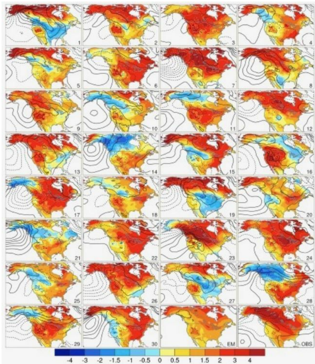
Bild 1: Beispiel für deterministisches Chaos bei der Klimamodellierung Clara Deser et al. 2016, Journal of Climate 29: 2237-2258 © American Meteorological Society. Used with permission. Dargestellt sind die Ergebnisse von dreißig Simulationen des gleichen Klimamodells (Klima von Nordamerika im Winter) mit Anfangstemperaturen, die sich nur um einige 10^{-14} Grad Celsius unterscheiden. Sie ergeben, wie die Farbtemperaturen der verschiedenen Felder zeigen, sehr unterschiedliche Klimaprognosen, die zumeist nicht den Beobachtungen entsprechen. Rechts unten Feld EM: Mittelwerte, Feld OBS: Beobachtungen.
